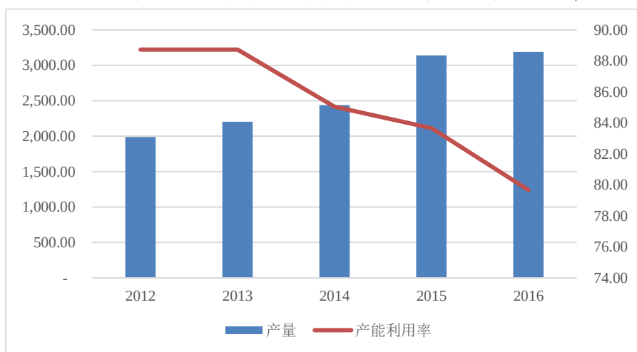
图 3 近年来我国电解铝产量及年平均产能利用率情况（单位：万吨，%）
