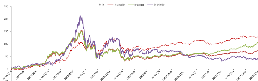
图表 17：组合历史收益曲线
